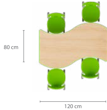
■ Wavy Table 120 x 80 cm
